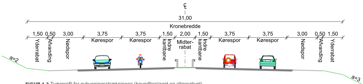
FIGUR 1.3 Tværprofil for nybygningsstrækningen (hovedforslaget og alternativet).
