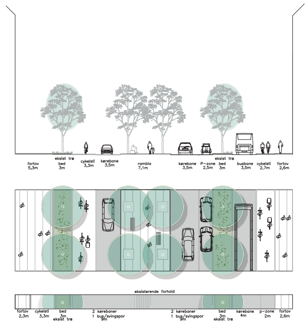
Figur 26: Principsnit og plantegning for en mulig fremtidig udformning af Holmens Kanal. Tegninger: LYTT Architecture
