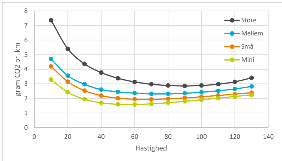
Figur 3: Sammenhængen mellem gennemsnitshastighed og CO 2 udledning pr. km for benzinerbiler med forskellig størrelse: store, mellem, små og minibiler, der lever op til EURO 5 og 6 normer (bilårsgange 2009-2019). Kilde den fælleseuropæiske COPERT-model.
